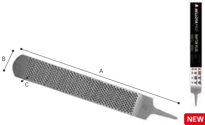
▶ РАШПИЛЬ 4140 RAPTOR PLUS
